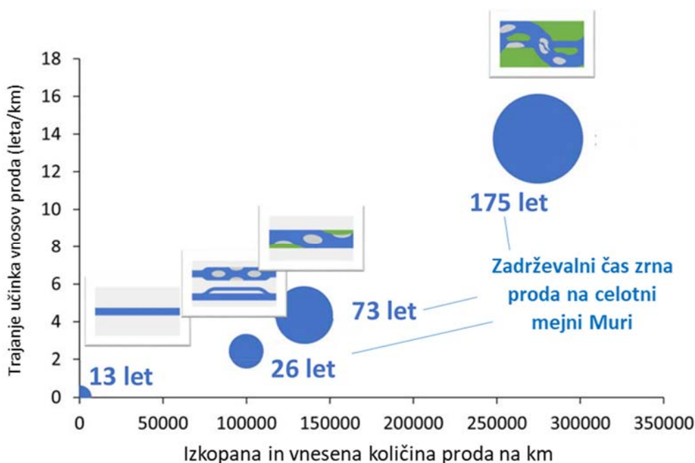
Slika 81. Učinkovitost rinjenih plavin različnih ukrepov, prikazana glede na trajanje učinka pridobljenega proda na tekoči kilometer različnih tipov ukrepov upošteva potreben vnos proda za odsek pri pripadajočem tipu ukrepa in glede na zadrževalni čas potujočega zrna proda na mejni Muri ob izvedbi pripadajočega tipa ukrepa na celotni mejni Muri.
