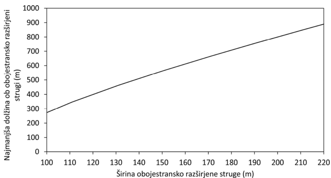
Slika 36. Izračunane najmanjše dolžine L_A odseka širitve na Muri za različne obsege širitve po Hunzingerju (1998). Upoštevati je treba, da šele najmanjše dolžine dopuščajo nastajanje morfologije v skladu s širino. Da potem ta morfologija prevladuje na večjem delu odseka, je treba omogočiti večje dolžine (npr. 2 \times L_A ).
