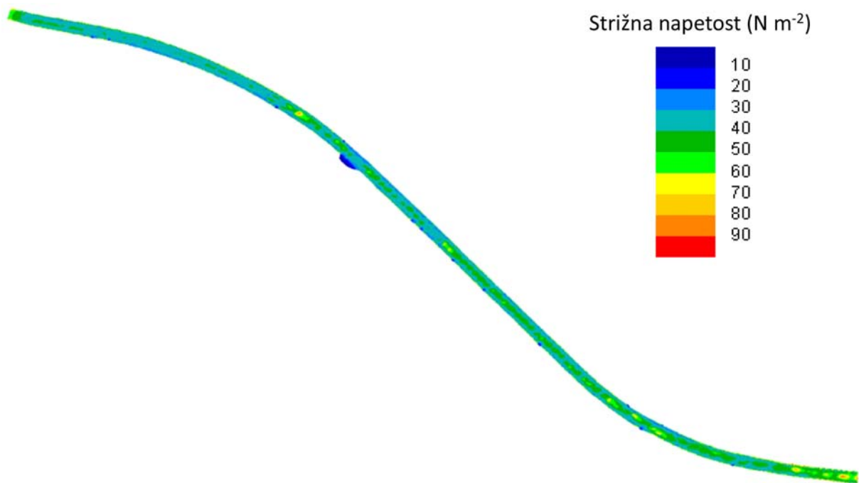
Slika 60. Strižne napetosti pretoka enoletne poplave v trenutni morfologiji referenčnega odseka
