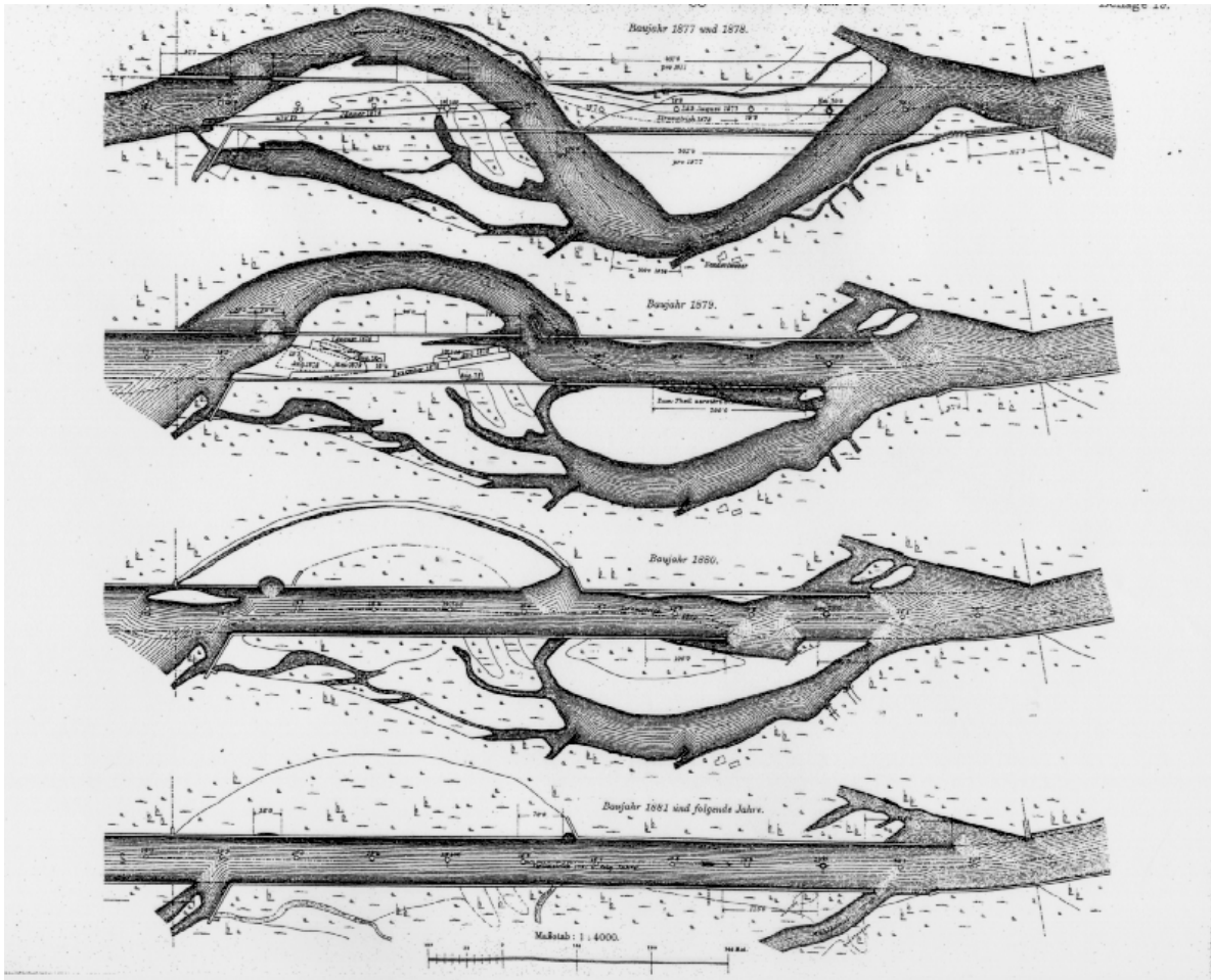
Slika 4. Časovni potek preboja od leta 1879 do 1881 v načrtih regulacije Hohenburger (po Habersack et al., 2001a)
