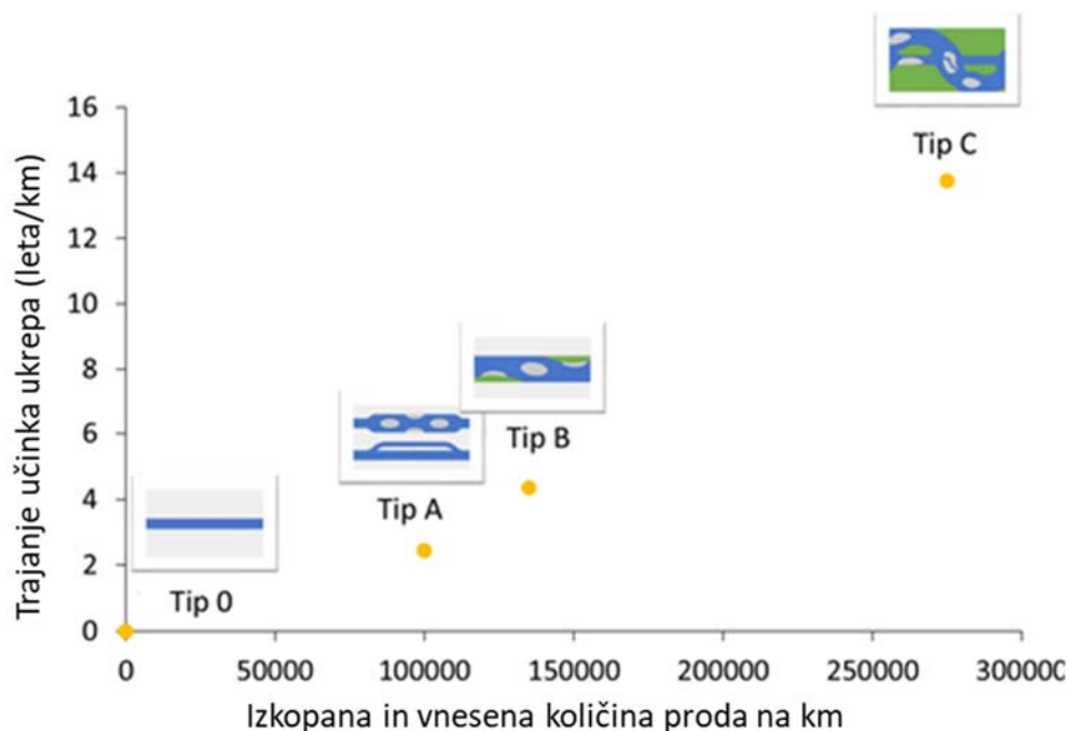
Slika 78. Trajanje učinka pridobljenega proda na tekoči kilometer različnih tipov ukrepov upošteva potreben vnos proda za odsek pri pripadajočem tipu ukrepa.
