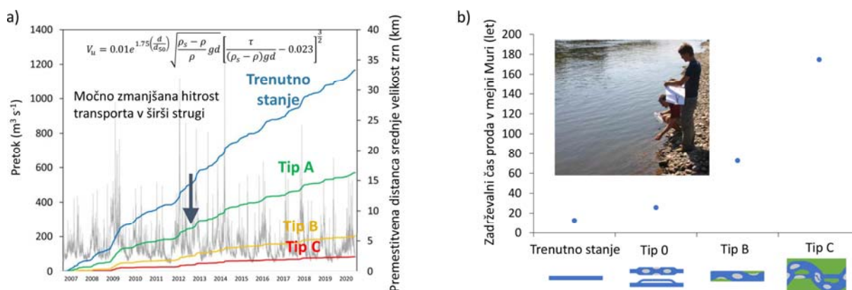
Slika 79. Zadrževalni čas rinjenih plavin v različnih tipih ukrepov
