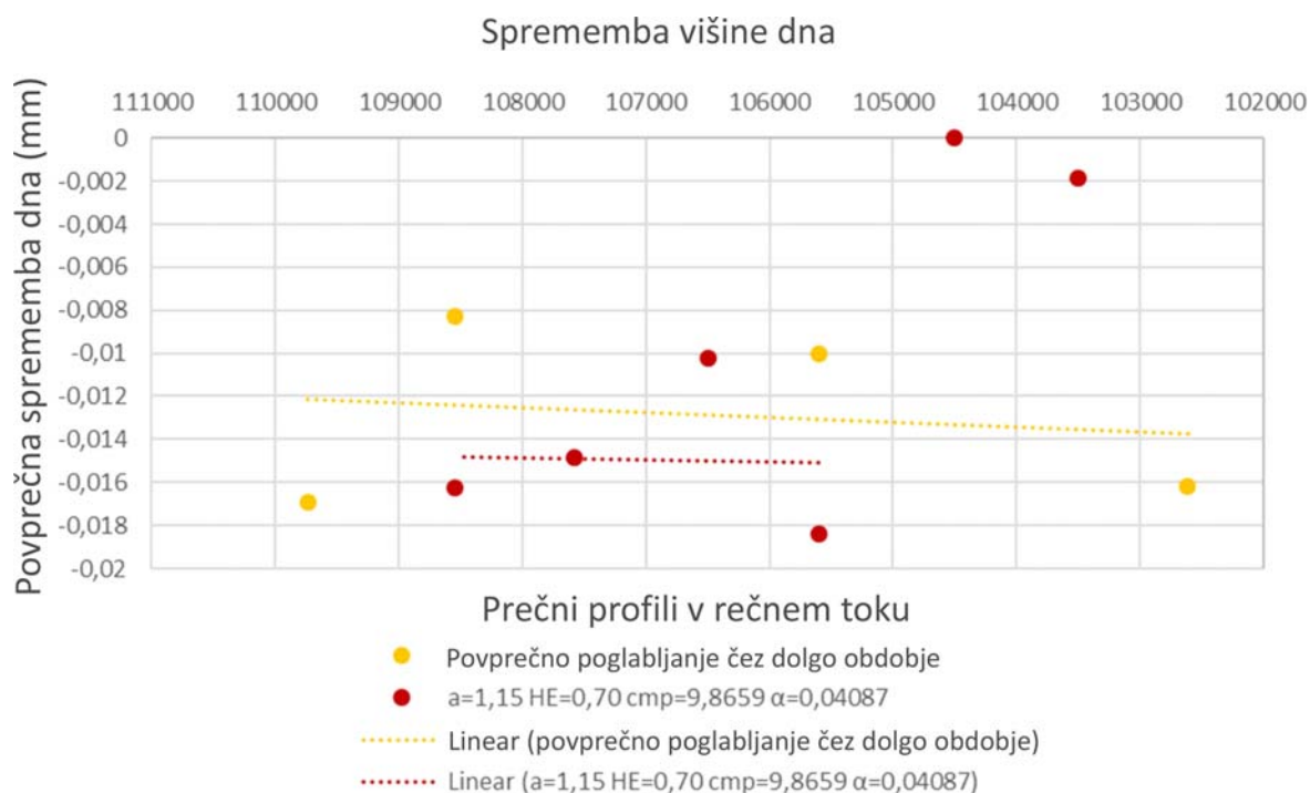
Slika 71. Rezultat umerjanja modela premeščanja rinjenih plavin, izvedenega na podlagi primerjave merjenih in modeliranih vrednosti poglobljanja
