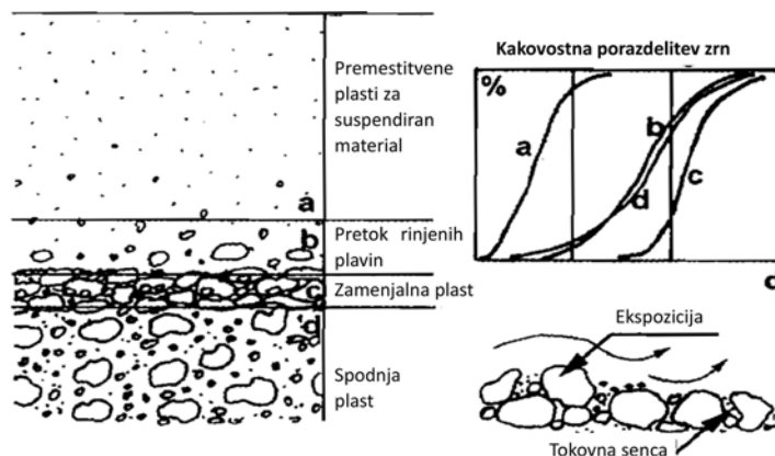
Slika 45. Struktura rečnega dna z zamenjalno plastjo (po ATV-DVWK, 2003)
