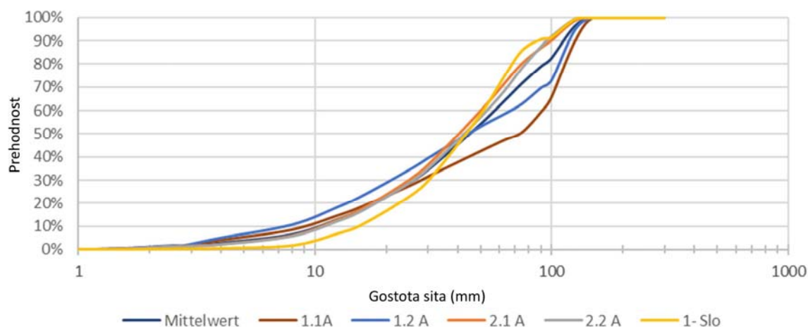
Slika 52. Zrnastostno razvrščanje z analizo linijskega vzorca plavin za ocenjevanje vrhnjega sloja tipa 0 v projektu mejna Mura
