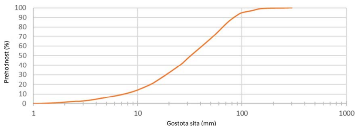
Slika 51. Zrnastostno razvrščanje v strugi iz volumskih vzorcev, ki smo jih vzeli v okviru Načelne vodnogospodarske zasnove za mejno Muro.
