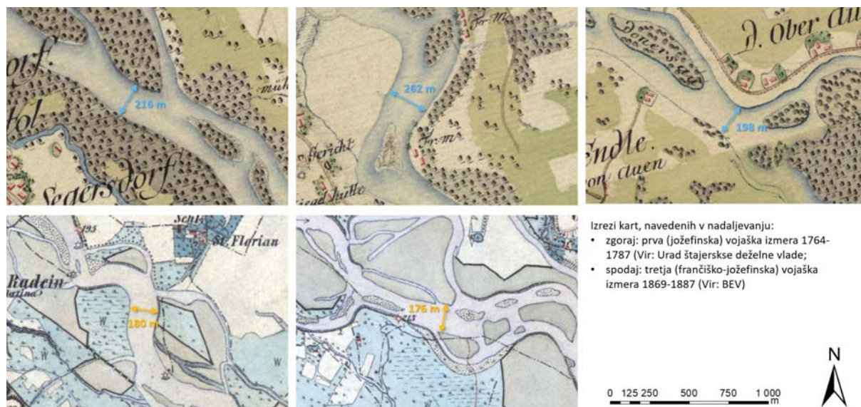
Slika 28. Oseki na zgodovinskih kartah odseka mejne Mure (slika levo spodaj se nanaša na stanje dolvodno od mejne Mure pri Radencih) z velikimi širinami stalno omočene struge
