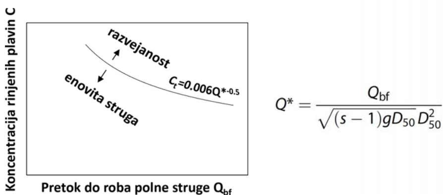
Slika 27. Odvisnost morfologije od koncentracije rinjenih plavin po Muellerju in Pitlicku (2014). Q_{bf} je pretočnost (pretok do roba struge), Q^* je brezdimenzijski pretok, s = je specifična gostota sedimenta ( \rho_s/\rho ) in D_{50} je mediana premera zrn. Koncentracija rinjenih plavin C se izračuna iz relacije med volumenskim premeščanjem rinjenih plavin ob pretoku do roba polne struge in pretokom polne struge. C_t je koncentracija rinjenih plavin na prehodu med strugo z enim in več rokavi.
