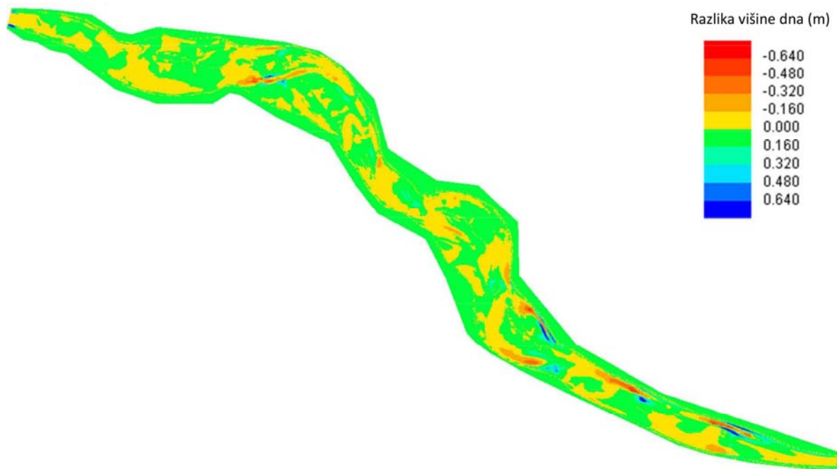
Slika 77. Morfodinamika pri tipu C po izračunu diagrama pretoka leta 1986
