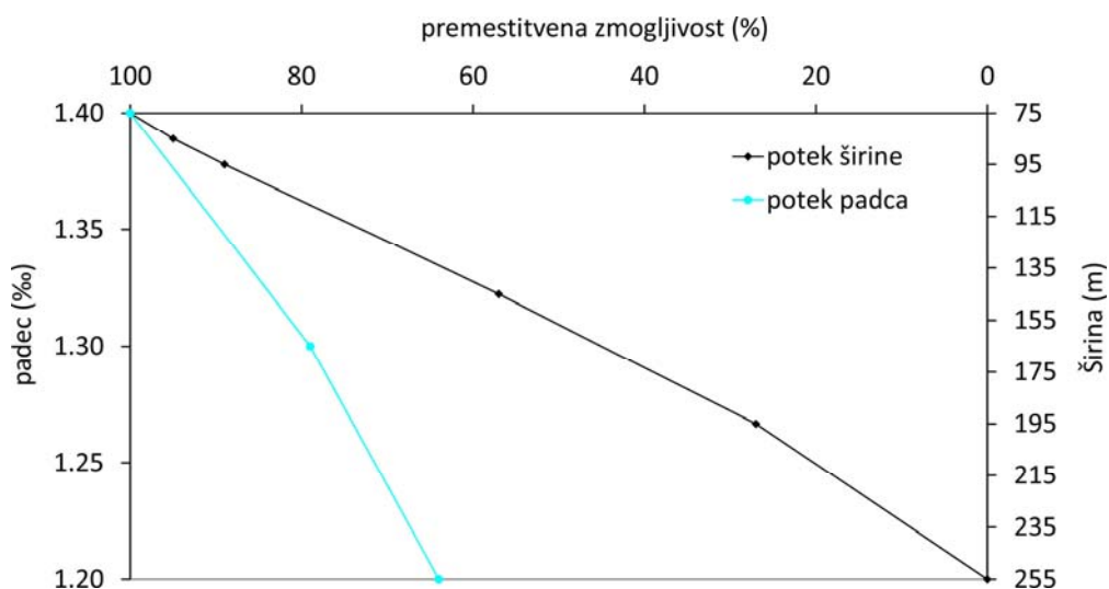
Slika 34. Odvisnost premestitvene zmogljivosti od padca in širine mejne Mure (po Habersacku in Schneiderju, 2000).
